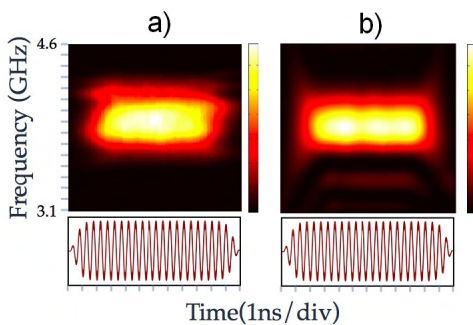
Figura 5: Espectrograma experimental (a) y obtenido con la formulación propuesta (b) de un pulso temporal cuadrado.
