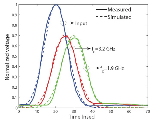
Figura 1: Propagación de pulsos temporales Gaussianos en una línea de transmisión CRLH [1]. Comparación de la formulación propuesta con medidas experimentales.
