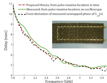
Figura 2: Retardo de grupo en función de la frecuencia obtenido con la formulación propuesta. Medidas experimentales son usadas como validación.
