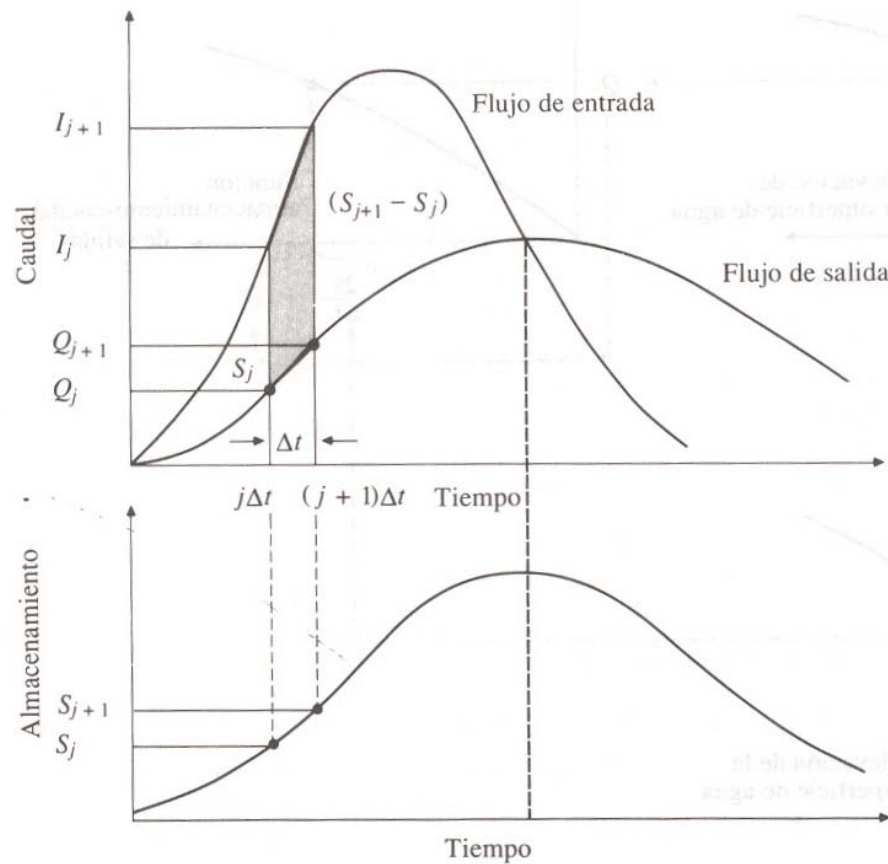
Figura 11. Cambio de almacenamiento durante un período de tránsito \Delta t .
