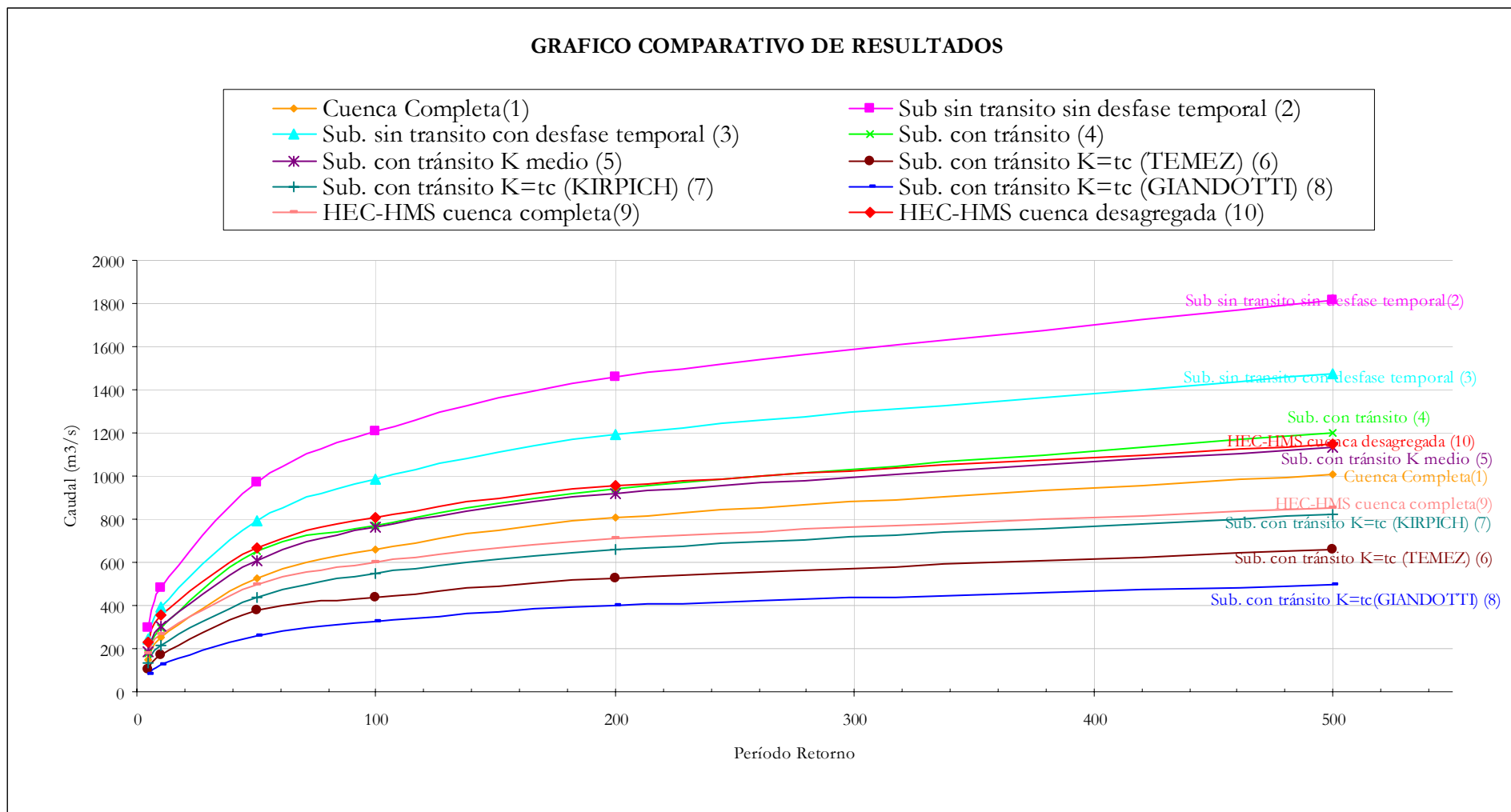
Figura 24. Gráfico comparativo de caudales para los distintos métodos de cálculo.
