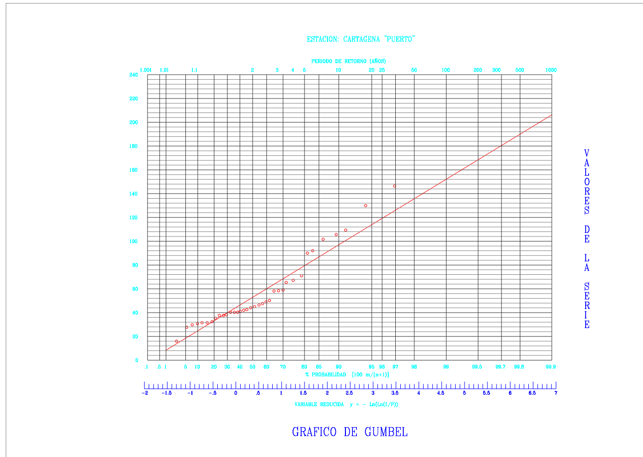
Figura 15. Ajuste probabilístico de Gumbel
