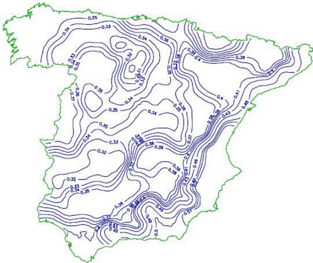
Figura 8. Isolíneas del valor regional del coeficiente de variación C_v .
