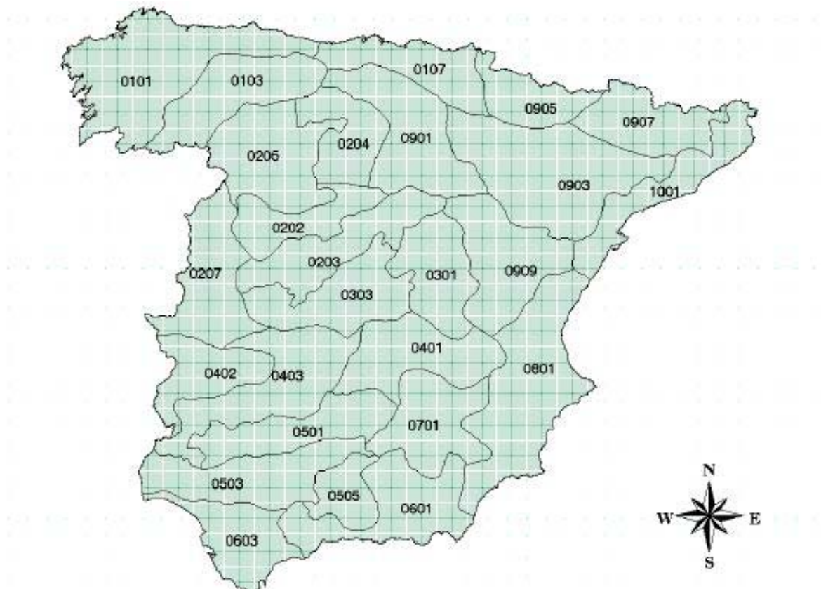
Figura 7. División de la España Peninsular en 26 regiones con características meteorológicas comunes.
