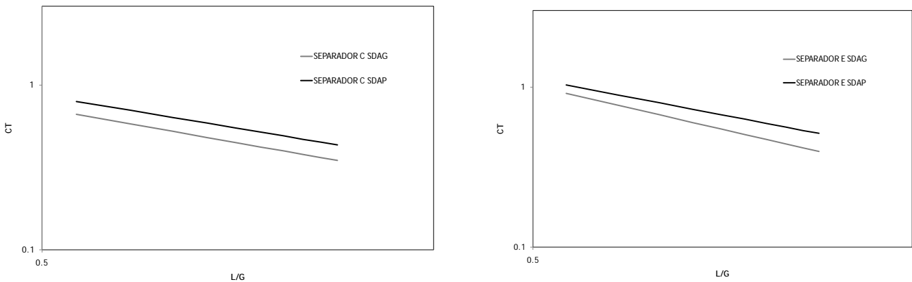
Figura 8: Comparativa de los separadores de gotas C y E con los sistemas por gravedad y presión respectivamente.
