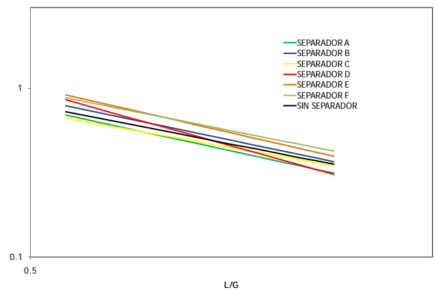
Figura 7: Correlaciones para los seis separadores de gotas ensayados más el caso sin separador para el SDAG.
