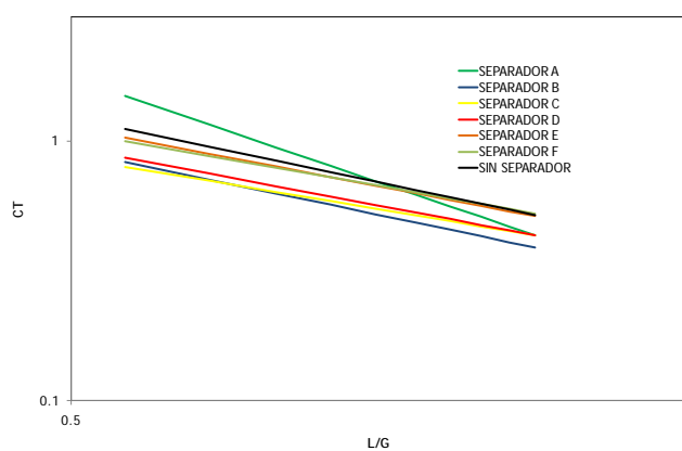
Figura 6: Resultados obtenidos por Lucas et al. (2009) incluyendo correlación obtenida cuando no hay separador de gotas.
