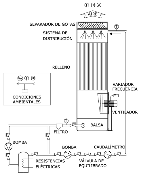
Figura 2: Diagrama esquemático de la instalación experimental.
