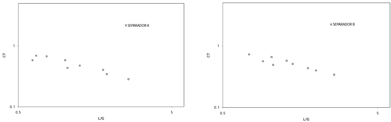
Figura 5: Característica Térmica frente a ratio caudales máxicos agua-aire para los separadores ensayados con el SDAG.
