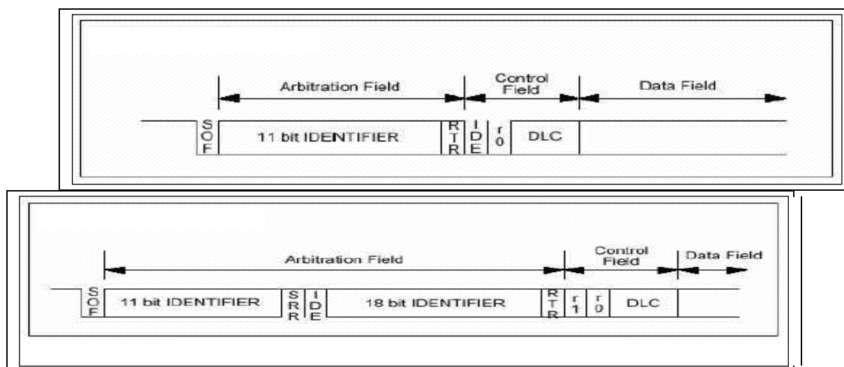
Figura 3.21.- Trama de datos estándar (arriba) y trama de datos extendida (abajo)
