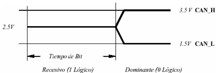
Figura 3.17.-Niveles eléctricos del bus CAN
