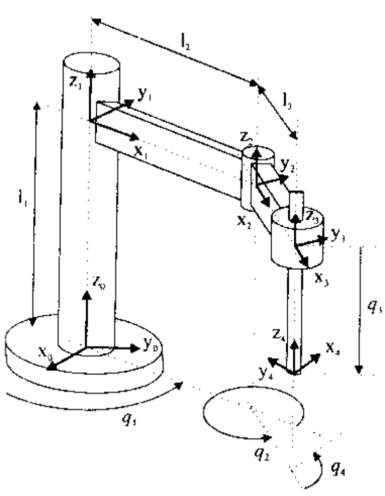
Figura 3.11.- Muestra de un brazo robótico con diferentes ejes de coordenadas
