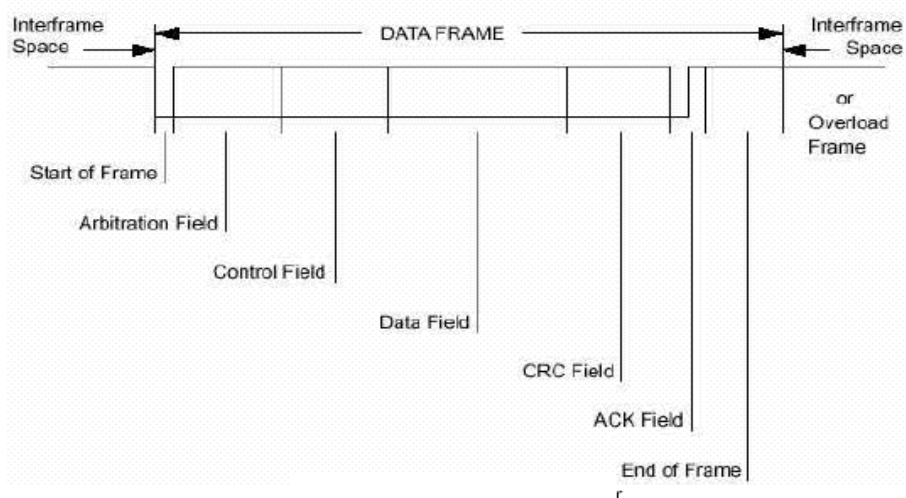
Figura 3.19.-Trama de datos estándar
