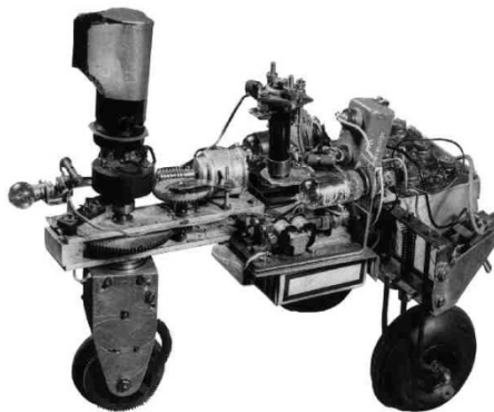
Fig.2.2: Foto Robot ELSIE.
