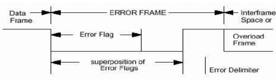
Figura 3.22.- Trama de error
