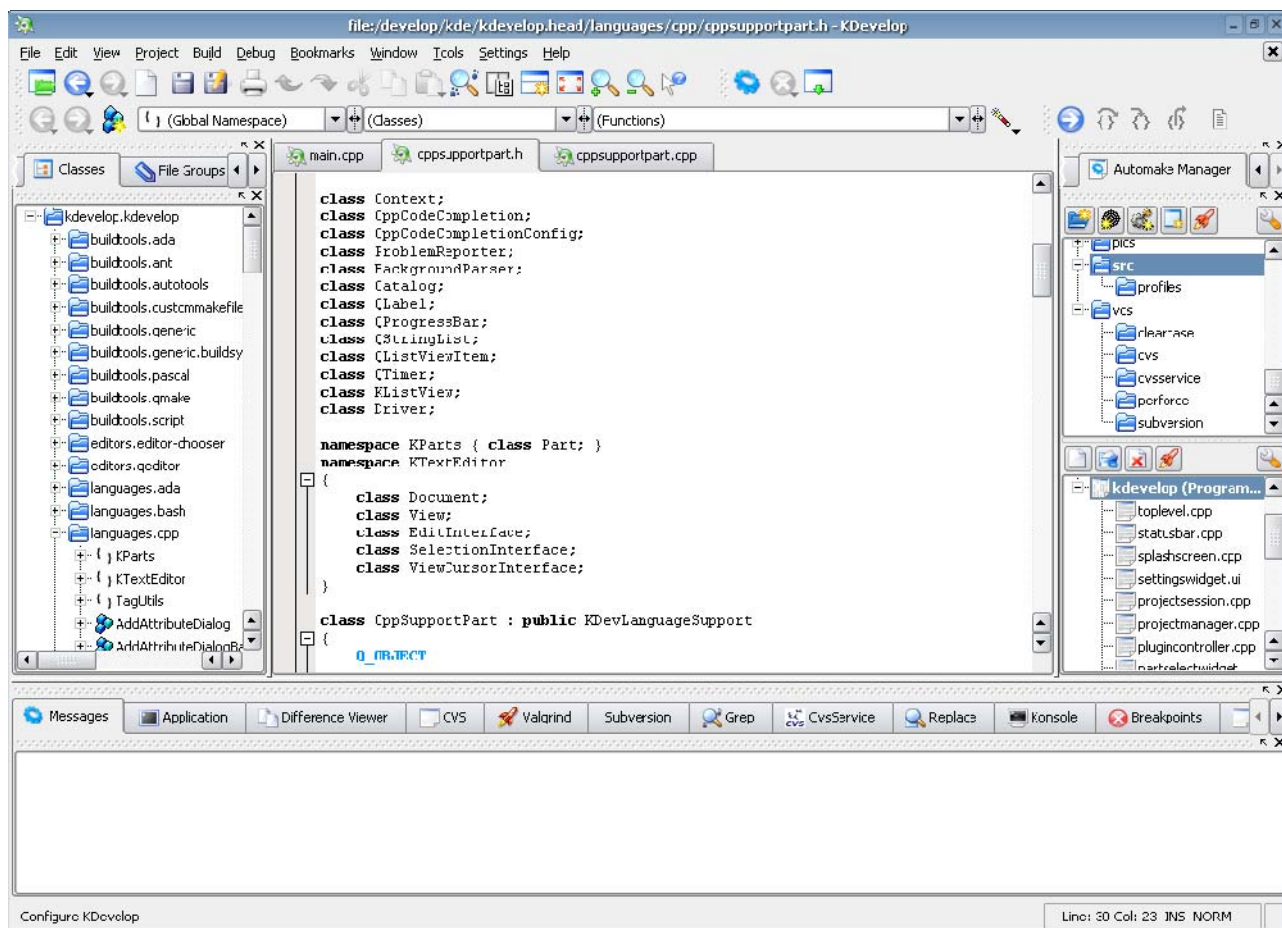
Fig.4.11.- Entorno Kdevelop
