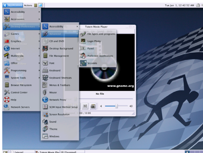
Fig. 4.7.- Escritorio GNOME
