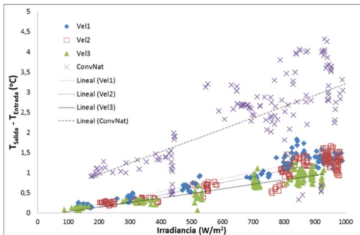
Figura 4: Datos experimentales de diferencia de temperatura entre entrada y salida para diferentes velocidades con b/L=0,0825 .
