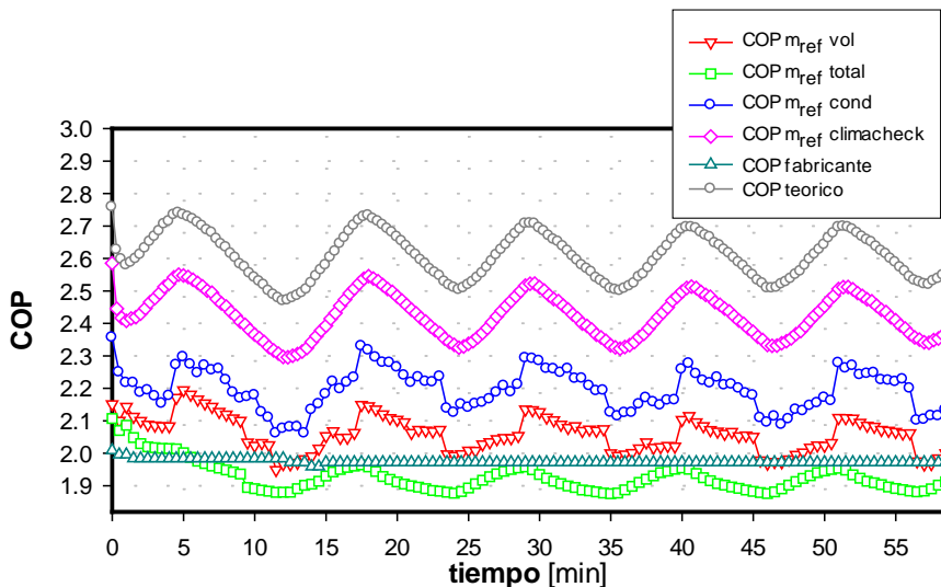
Figura 12. COP en el experimento cuasiestacionario.
