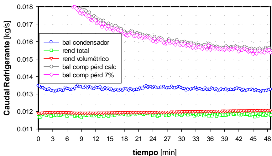
Figura 10. Predicción del caudal de refrigerante en el experimento con carga de 1000 W constante.
