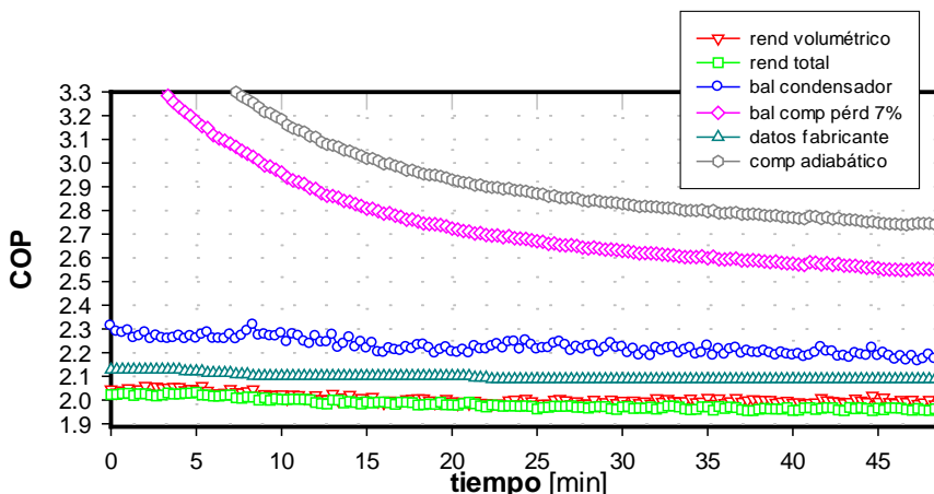
Figura 11. Predicción del COP en el experimento con carga de 1000W constante.
