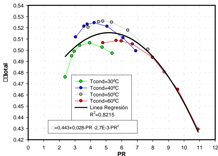
Figura 7. Ajuste del rendimiento total con la relación de compresión, para el compresor Tecumseh CAJ9510Z, a partir de datos tabulados proporcionados por el fabricante.
