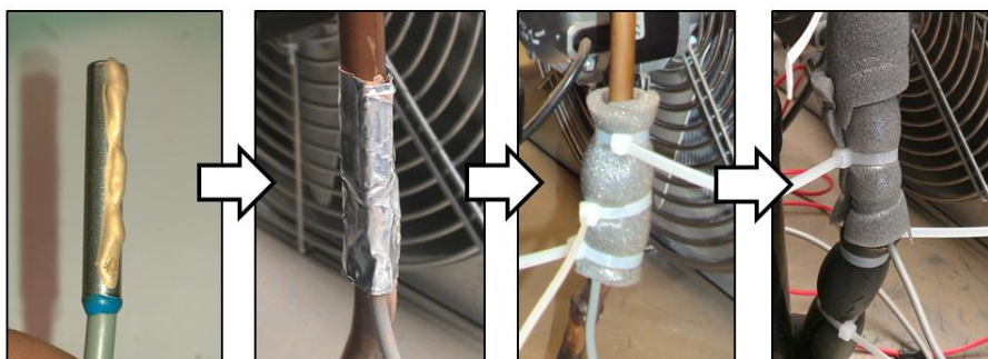
Figura 8. Método experimental para medir la temperatura en el circuito frigorífico. De izquierda a derecha: pasta térmica, cinta de aluminio, aislante sobre la sonda, aislante en el entorno de la sonda para evitar minimizar efectos de conducción a lo largo de la tubería de cobre.
