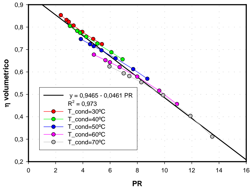
Figura 6: Ajuste lineal del rendimiento volumétrico con la relación de compresión, para el compresor Tecumseh CAJ9510Z, utilizado en la cámara frigorífica estudiada, a partir de datos del fabricante.
