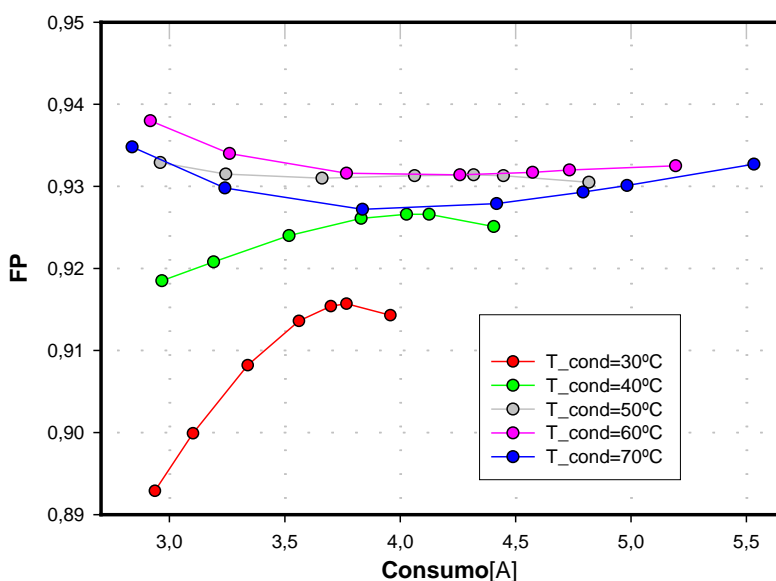
Figura 9. Factor de potencia en función de la intensidad consumida y de la temperatura de condensación del compresor Tecumseh CAJ9510Z, elaborado a partir de datos del fabricante.
