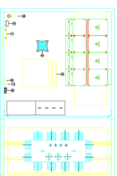
PLANTA
