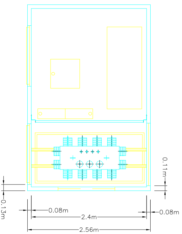
PLANTA
