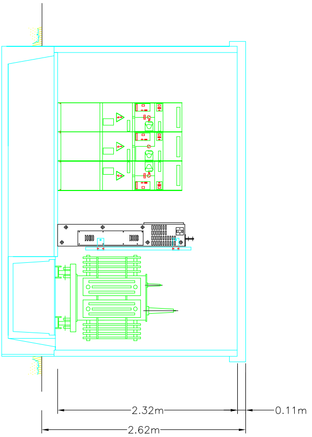
ALZADO
