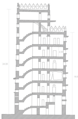
Fig. 2. Sección tipo de casa torre. Elaboración propia a partir de Ortega (2008).
