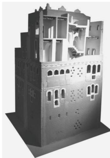
Fig. 6. Maqueta de casa-torre de Yemen. Imagen del autor obtenida en la Exposición "Learning from vernacular" de Arquería de Nuevos Ministerios, Madrid, 2011.
