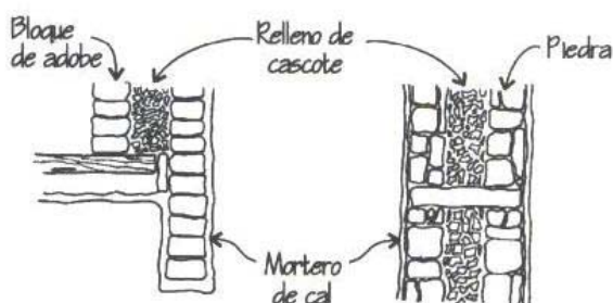
Fig. 5. Sección vertical del muro de carga de la casa-torre. A la izquierda, muro de adobe en encuentro con forjado y formación de hueco en pisos superiores; a la derecha, sección de muro de piedra en planta baja (Neila González, 2004).
