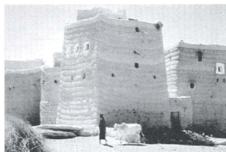
Fig. 4. Vivienda de varios pisos usando la técnica zabur (Gernot, 2001).
