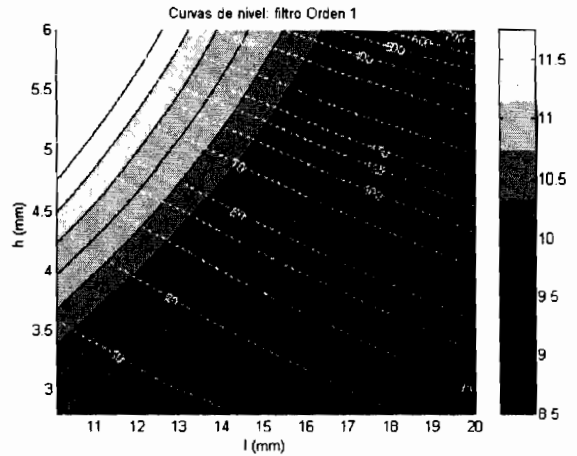
Fig2: Curvas de nivel para un único resonador.
