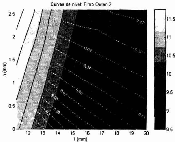
Fig3: Curvas de nivel para dos resonadores acoplados.
