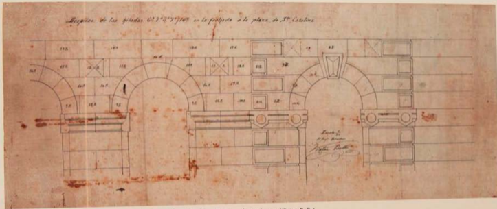
Plano de despiece de la fachada Oeste del Palacio Consistorial realizada y firmada por Víctor Beltrí
