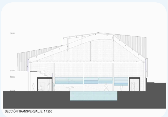
Plano de la sección transversal de la Piscina Cubierta
