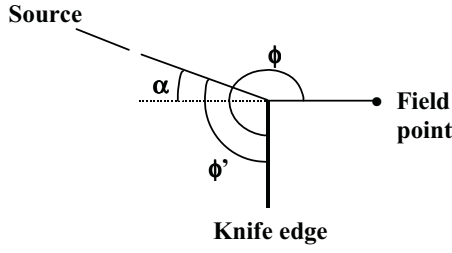
Fig. 2. Descripción de la geometría correspondiente a la difracción en un knife edge .
