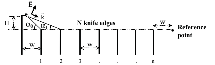
Fig. 1. Esquema del entorno de propagación considerado, en el que se aprecia la fuente emisora y la serie de láminas semi-infinitas.
