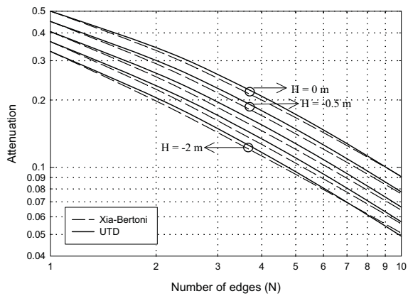
Fig. 4. Atenuación en función de la altura de la antena emisora para distintos valores de N (número de láminas). Se ha considerado H \leq 0 ( 0_m \leq 0 ).
