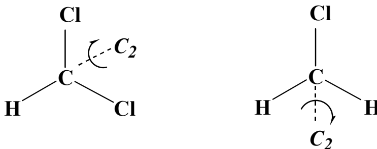
Figura 12. -Molécula CH_2Cl_2 , vista desde el enlace C–H y C–Cl (se omiten H y Cl respectivamente)
