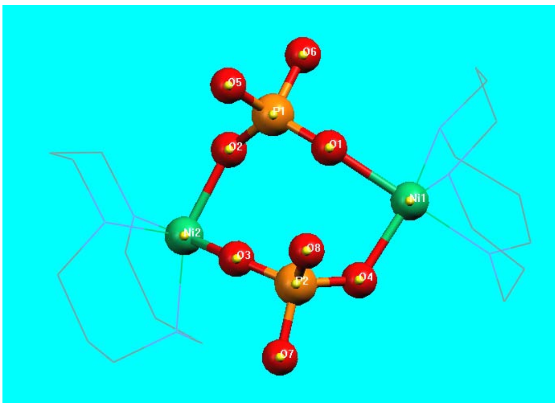
Figura 1.- Estructura (parcial) del catión del complejo (a)
