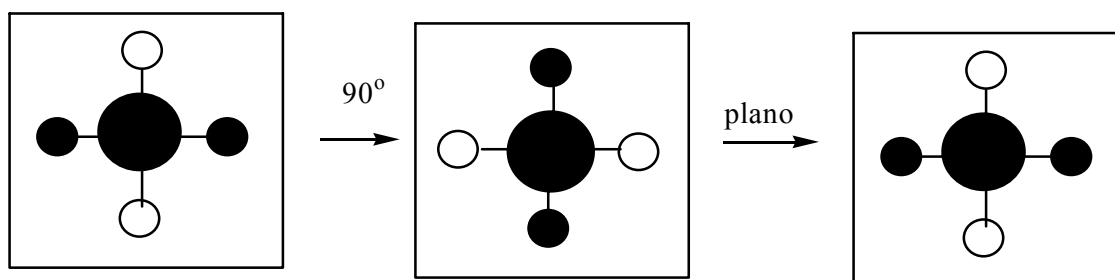
Figura 19.- Operación de simetría S_4 aplicada al \text{CH}_4
