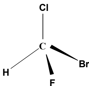
Figura 9.- Molécula \text{CHFClBr}
