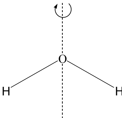
Figura 4.- Molécula de agua, H 2 O
