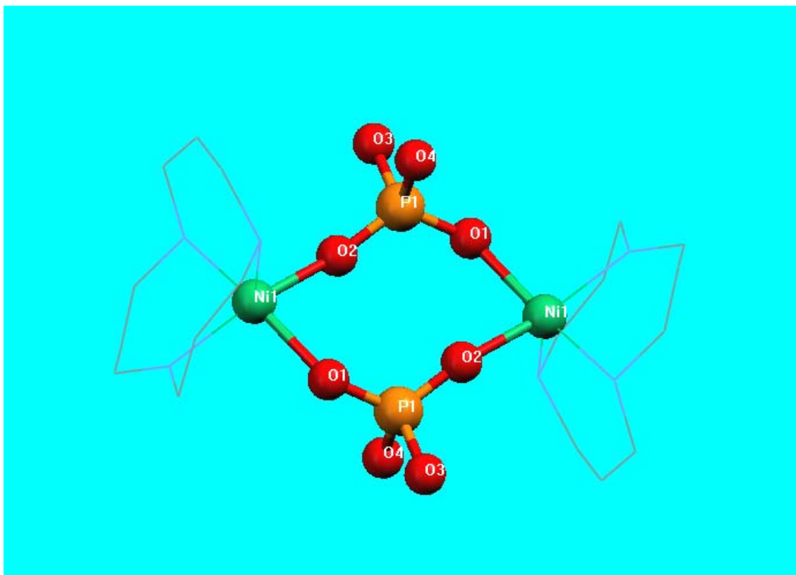
Figura 2.- Estructura (parcial) del catión del complejo (b)
