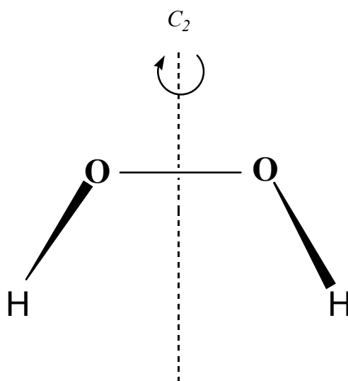
Figura 11.- Molécula H_2O_2
