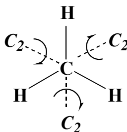
Figura 7.- Molécula \text{CH}_4 vista desde uno de los enlaces C-H (se omite el H por claridad)
