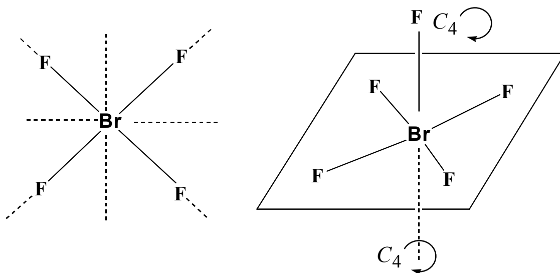
Figura 14.- Molécula de \text{BrF}_5
