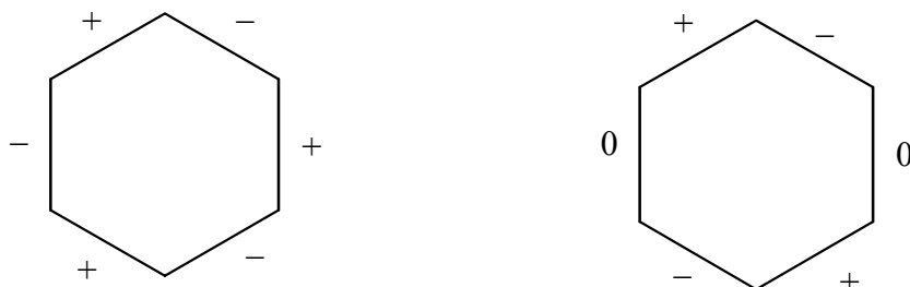
Figura 25.- Representación de signos de las configuraciones chair y boat del ciclohexano
