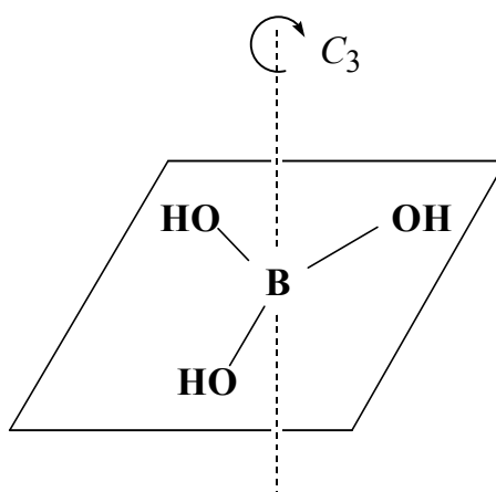
Figura 16.- Molécula de ácido bórico
