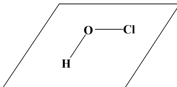
Figura 10.- Molécula \text{HOCl}
