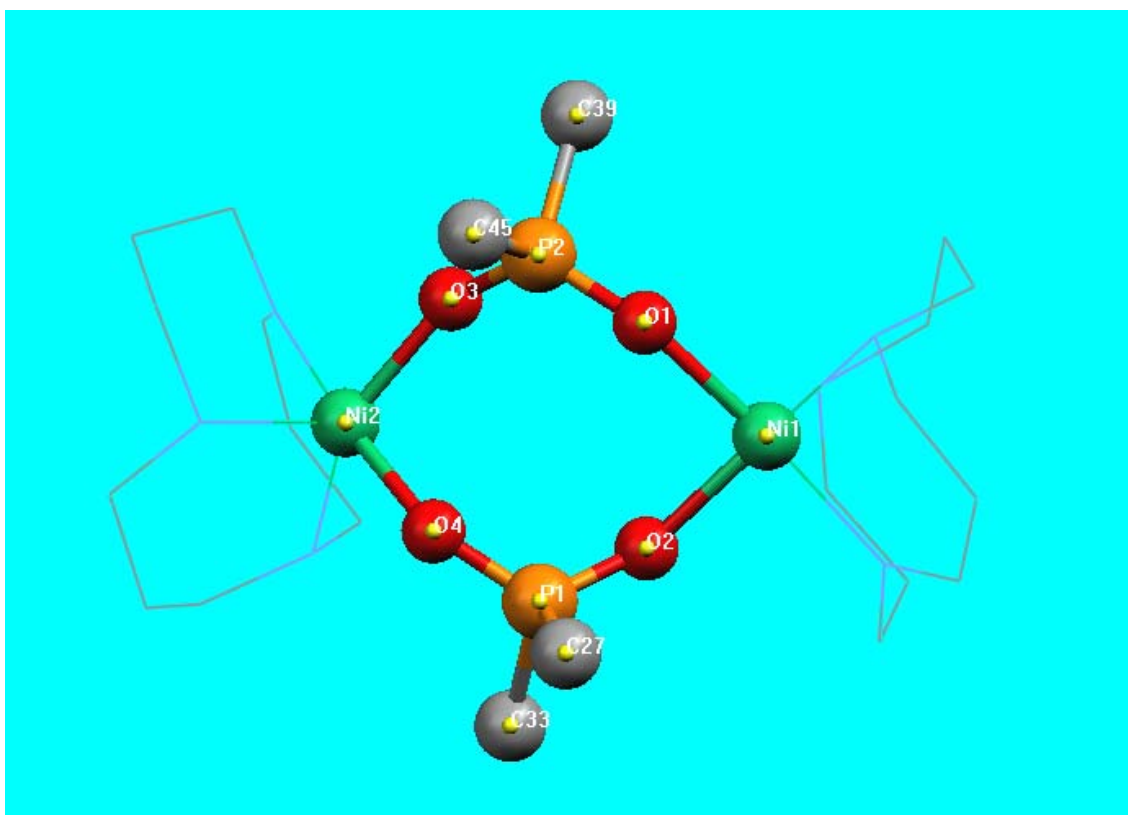
Figura 3.- Estructura (parcial) del catión del complejo (c)
