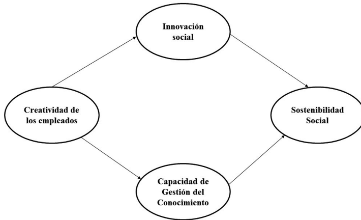
Figura 4. Modelo propuesto
