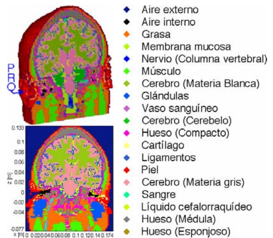
Fig. 1. Plano coronal del modelo de cabeza del Proyecto Humano Visible.
