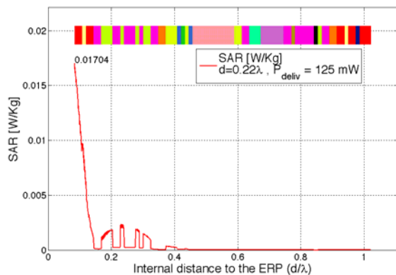
Fig. 5. TAE para los tejidos encontrados desde el PRO (a 0.22 \lambda del dipolo).
