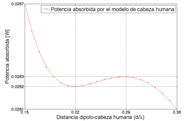
Fig. 2. Potencia absorbida en función de la distancia dipolo-cabeza.
