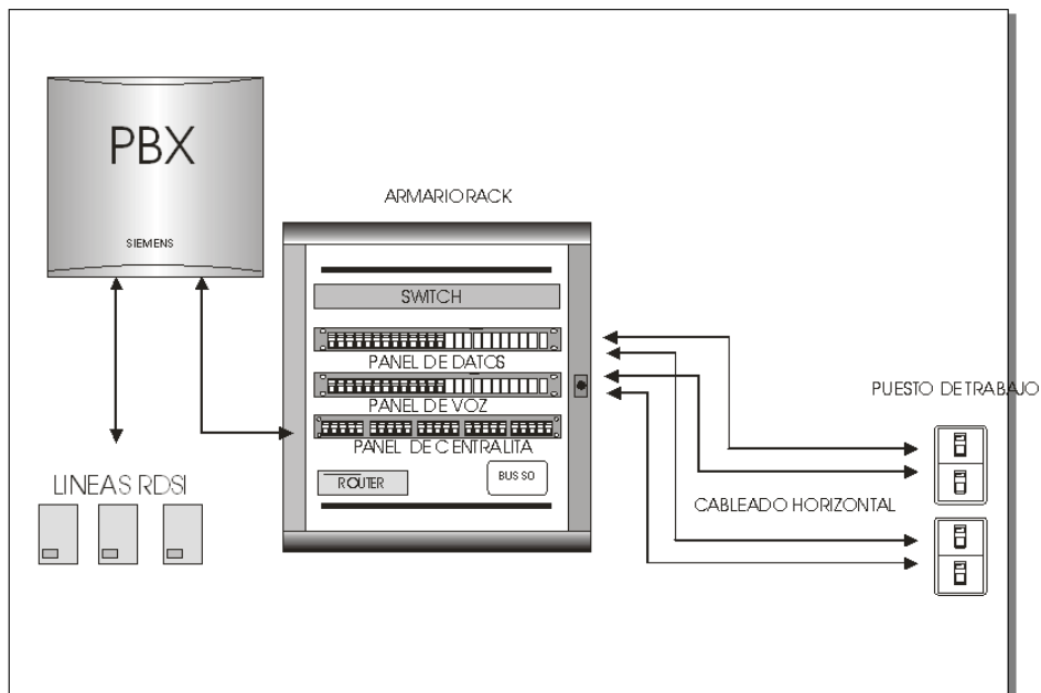
Figura 3. 1 Esquema de acometida celda de operador
