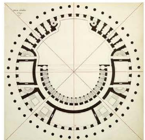
[6] ÉTIENNE-LOUIS BOULLEE, [BNF] «PROJET DE OPÉRA AU CARROUSEL», 1781. PLANTA DEL ACCESO. [P+C]
