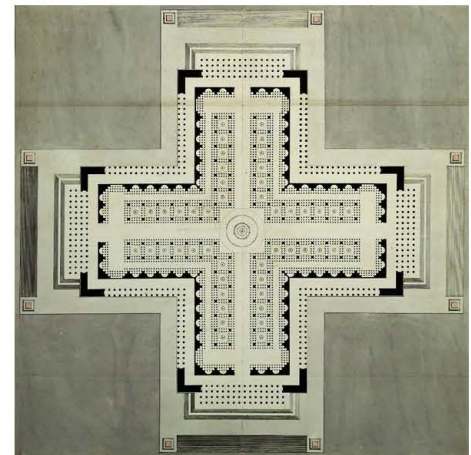
[14] ÉTIENNE-LOUIS BOULLEE, [BNF] «PROJET DE BASILIQUE A L'ÊTRE SUPREME», 1781. PLANTA. [P+C]
