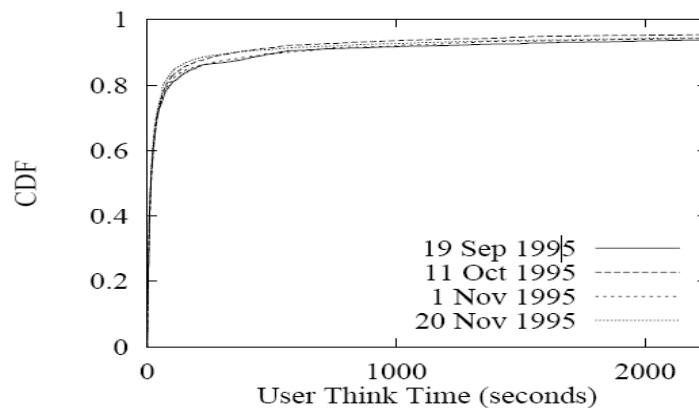
Fig. 2.7: FDP del tiempo de reflexión del usuario.
