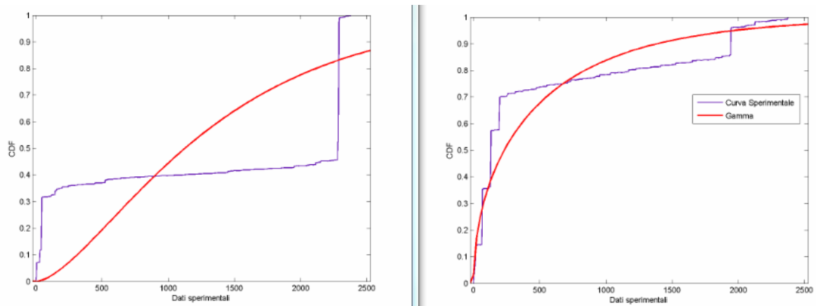
Fig. 5.5 : Modelización del Tiempo con Ajax y sin Ajax respectivamente
