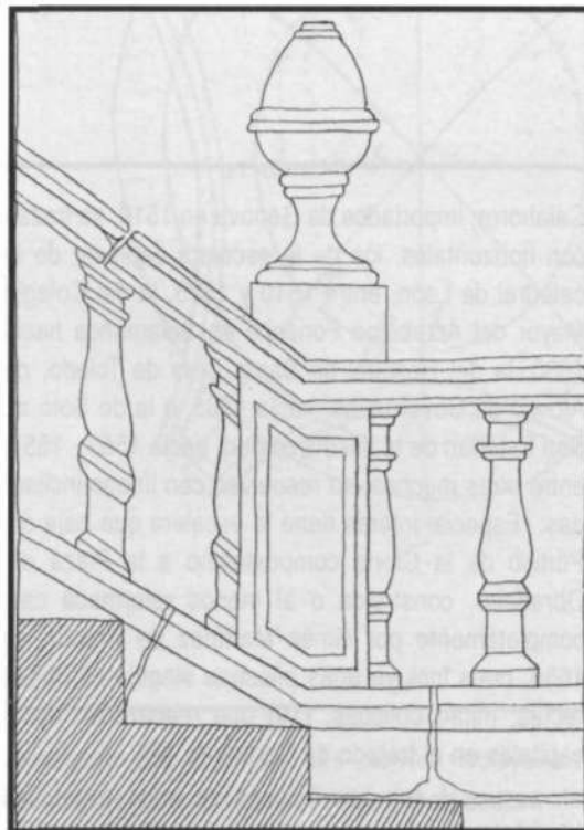
Balaustrés de la escalera del Obradoiro de la catedral de Santiago de Compostela. Ginés Martínez de Aranda 1608-1608. Dibujo del autor.
