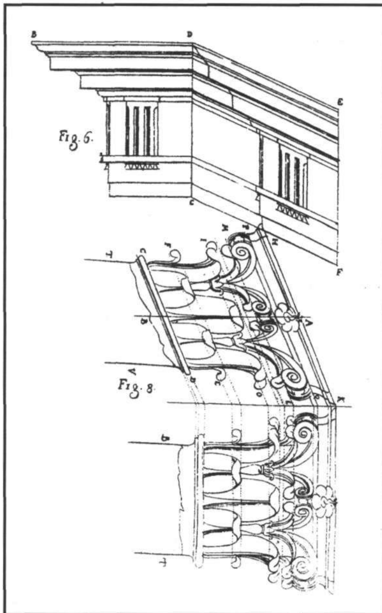
Frisos y capiteles oblicuos. Guarino Guarini. Architettura Civile , tratado III, lámina XV
