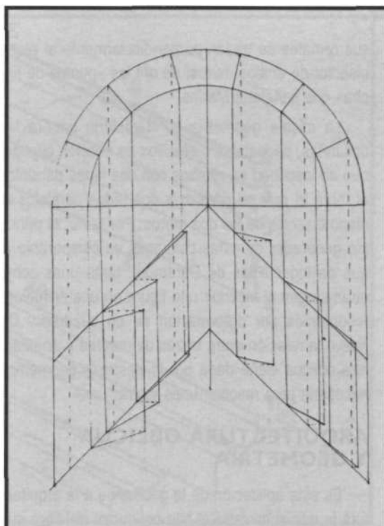
Ventana de ángulo en el palacio de los Guzmanes de León. Dibujo del autor.
