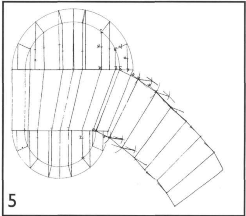
Arco en cuadrado y viaje. Alonso de Vandelvira. Libro de trazas y cortes de piedras , f 26 v
