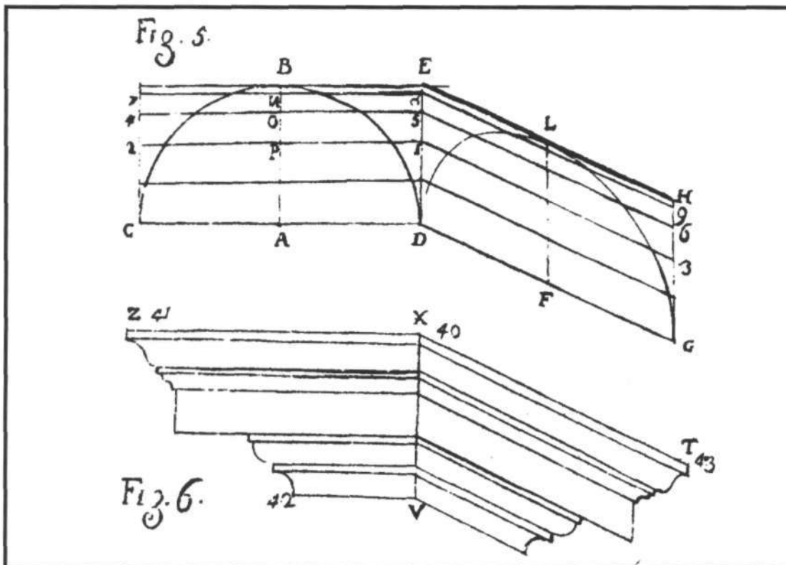
Cornisas oblicuas. Guarino Guarini. Architettura Civile , tratado III, lámina XV
