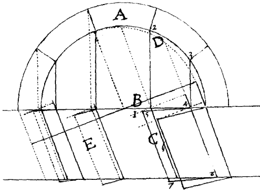
Figure 3 Ginés Marínez de Aranda. Cerramientos y trazas de montea , pl. 16. Arco en viaje por cara y por plantas
