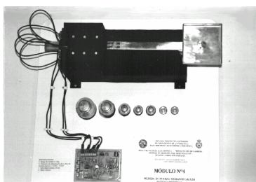
Figura 4: Equipo y diagrama de bloques para la medida de fuerza
