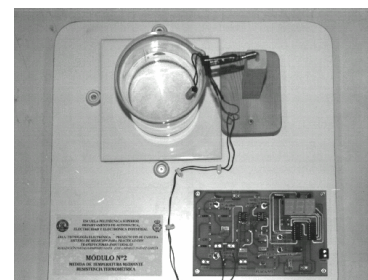
Figura 2: Disposición circuital y equipo para la medida de temperatura
