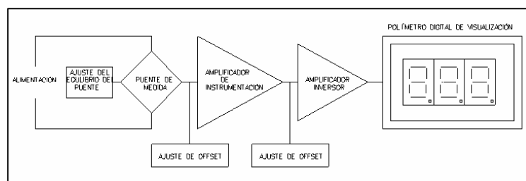
Figura 4: Equipo y diagrama de bloques para la medida de fuerza
