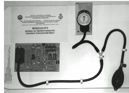
Figura 1: Disposición circuital y equipo para la medida de presión
