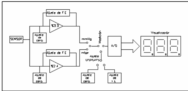
Figura 1: Disposición circuital y equipo para la medida de presión
