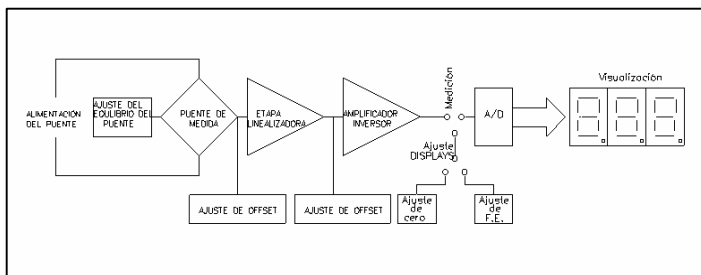
Figura 2: Disposición circuital y equipo para la medida de temperatura
