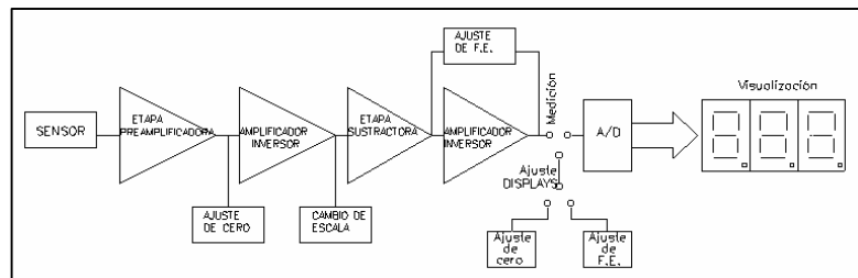
Figura 3: Equipo y disposición circuital para la medida de pH
