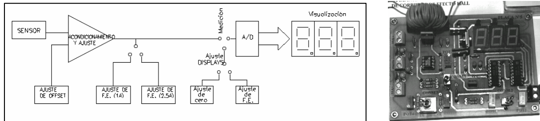
Figura 5: Equipo y diagrama de bloques para la medida de fuerza
