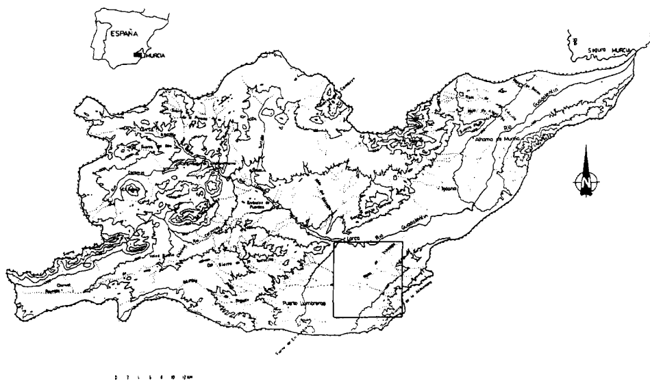
FIGURA 2. Localización general dentro de la cuenca del río Guadalentín.
