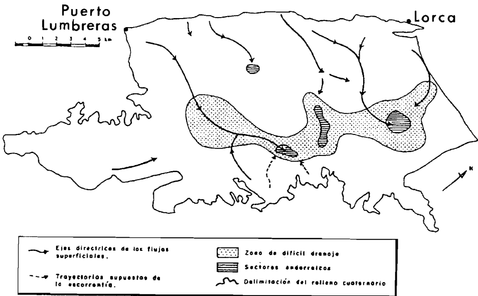
FIGURA 9. Trayectoria de los flujos superficiales en la base el Cuaternario (CONESA, SOLÍS, SÁNCHEZ Y CABEZAS, 1994).
