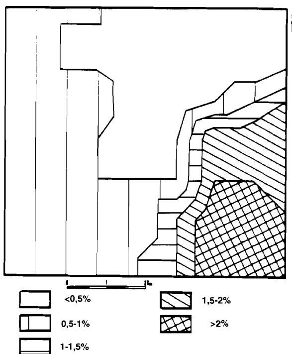
FIGURA 3. Mapa de pendientes.
