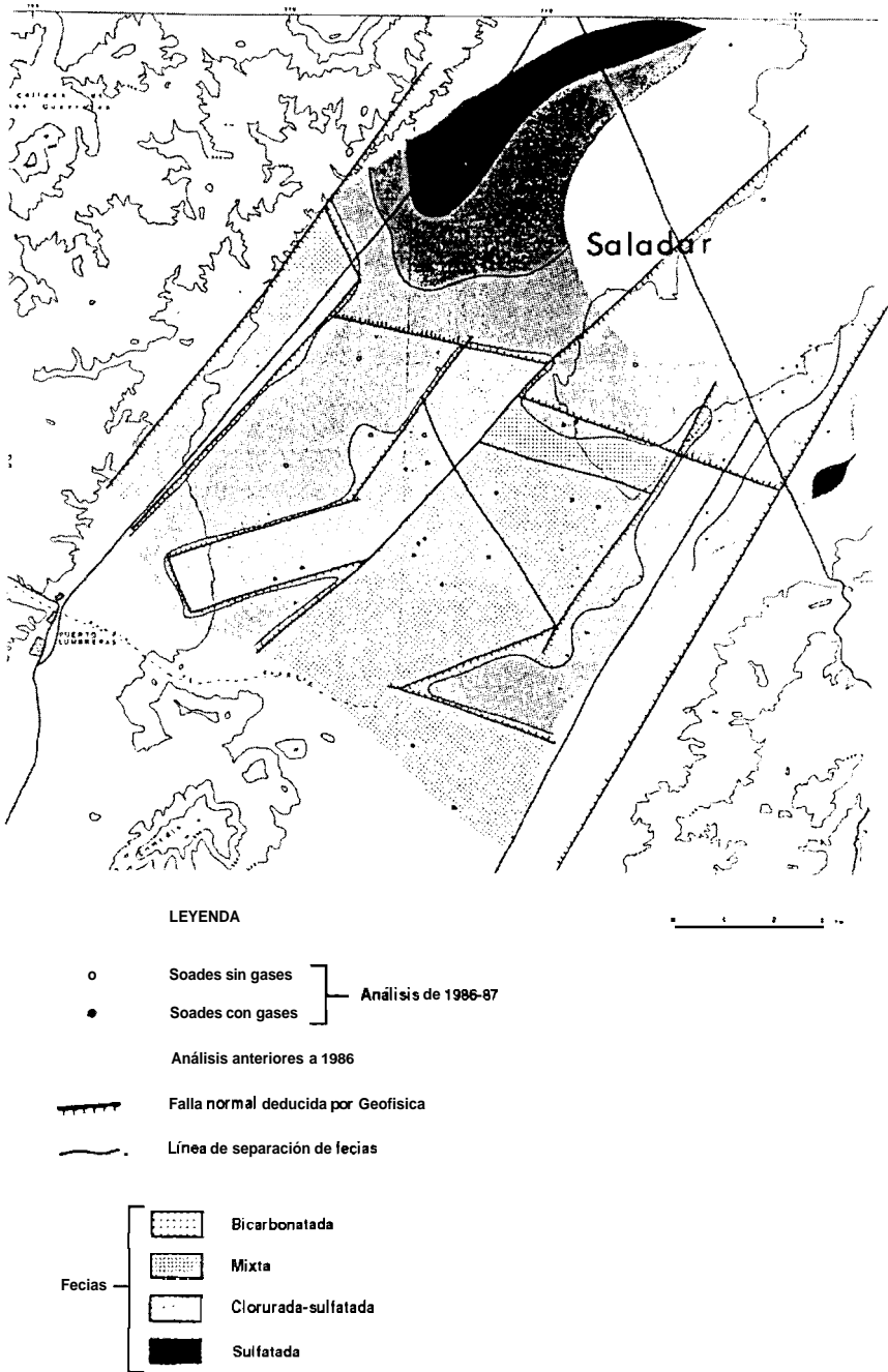
FIGURA 5. Estructura del zócalo en el Alto Guadalestín y facies químicas. (RODRÍGUEZ ESTRELLA, 1987)
