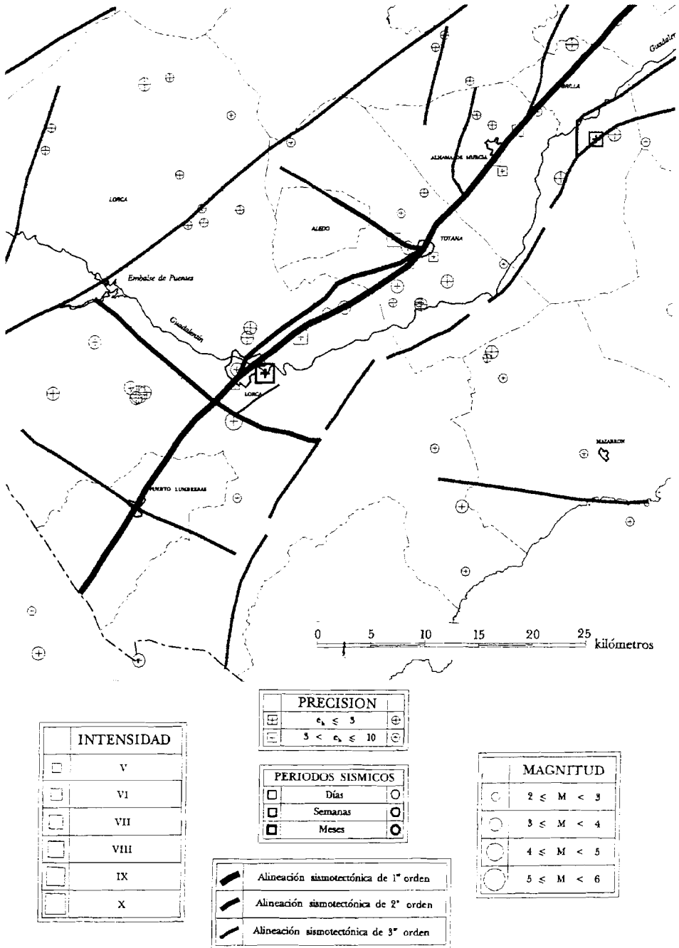
FIGURA 10. Mapa sismotectónico del Valle del Guadalentín y zonas adyacentes (IBARGÜEN Y RODRÍGUEZ ESTRELLA, en prensa).
