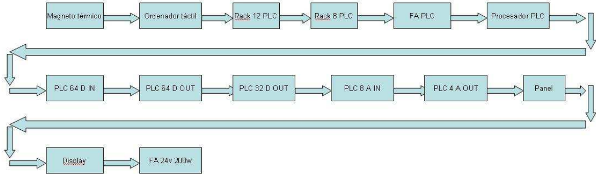
Figura 3. Diagrama funcional del Interface con el operador
